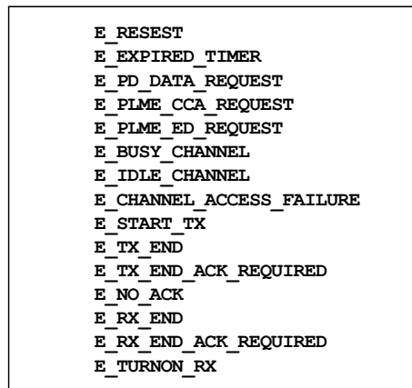
그림 5. TRx 이벤트 정의
