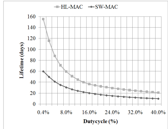
그림 10. 시스템 Lifetime 비교
