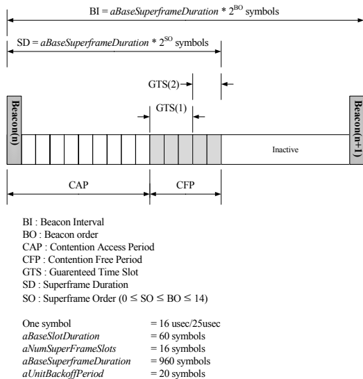
그림 2. IEEE 802.15.4 superframe 구조
