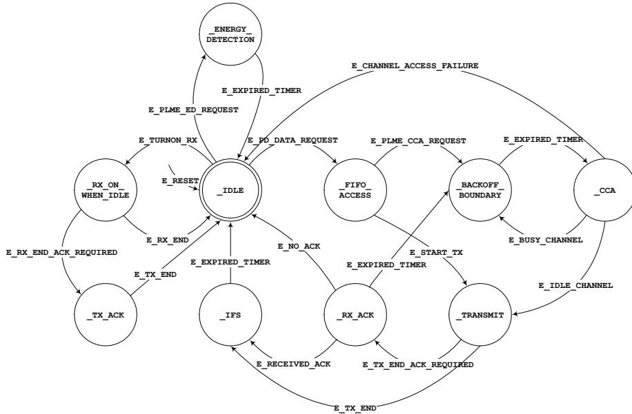
그림 6. 송수신 상태기계 다이어그램
