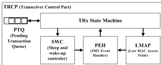
그림 4. 송수신기 제어부(TRCP)의 다이어그램
