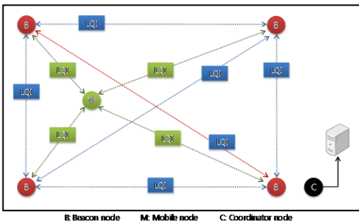
그림 2. 자가설정 위치추정 시스템의 전체적인 구성과 동작 방식에 대한 개념도
