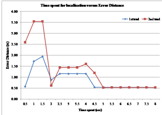
그림 8. 위치추정에 소요한 시간에 따른 위치추적 오차의 변화.
