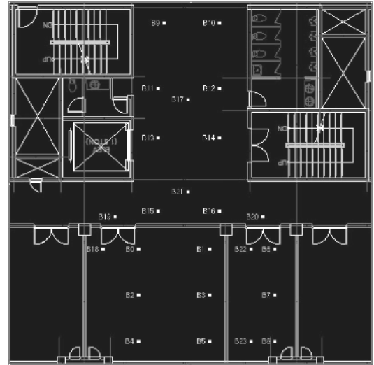
그림 5. 시험적으로 4층에 비콘노드를 배치한 예.
