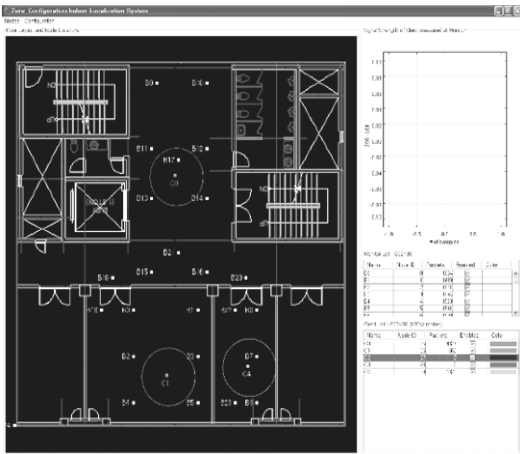
그림 4. 위치추적에 사용한 응용프로그램의 화면구성.
