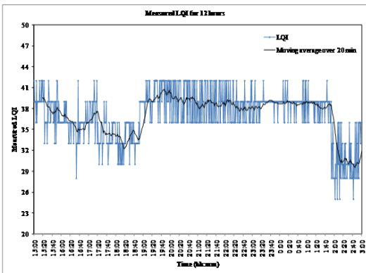
그림 6. 12시간에 걸쳐 1분 간격으로 측정한 5미터 떨어진 두 노드간 LQI값의 변화. 검은 실선은 20분 간격으로 LQI값에 대하여 이동 평균을 구한 결과이다.
