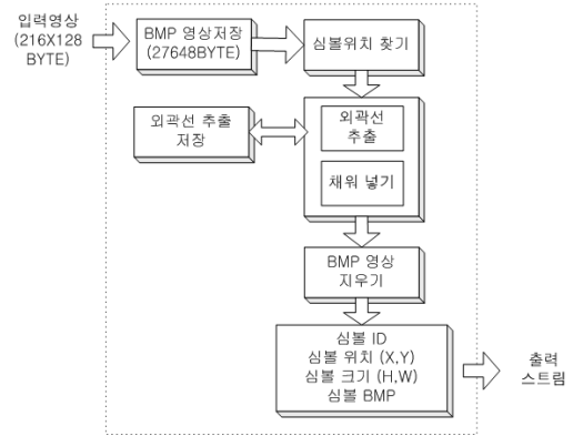
그림 2. 심벌 추출부의 구조
