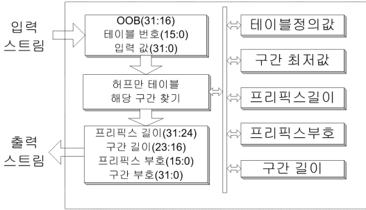
그림 3. 허프만 부호화기의 구조
