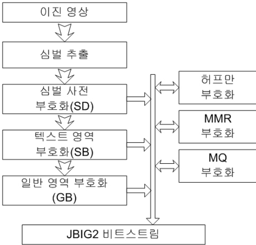
그림 1. JBIG2 부호기의 블록도
