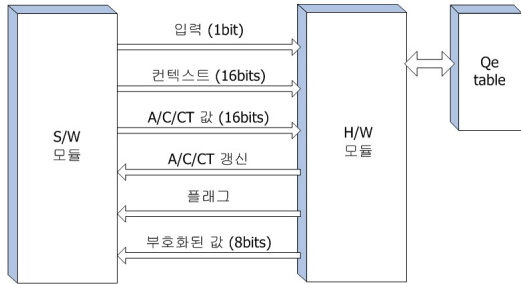
그림 5. MQ 산술부호화기의 소프트웨어 - 하드웨어 연동 설계 서 H/W 모듈의 B 레지스터의 값을 전송하거나 증가, 혹은 부호된 바이트를 전송하는지 S/W 모듈에 알려준다. 또한, 산술부호기의 속성상 입력이 인가된 후 출력이 발생하기까지는 불규칙한 지연이 발생한다. 따라서, 모든 입력이 완료가 된 후에도 하드웨어 모듈에는 가상입력을 계속 인가하여 최종 Byteout이 0xAC, 0xFF가 출력 되는 것을 확인한 후에 하드웨어 모듈을 종료시키도록 설계하였다.
