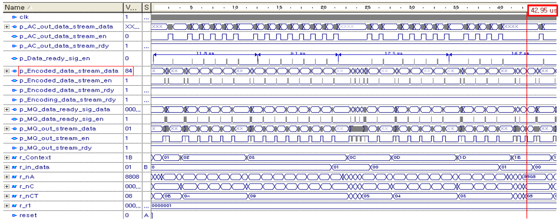
그림 9. MQ 산술부호화기 파형 검증 결과
