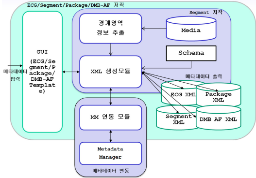
그림 5. DMB ECG 메타데이터 저작도구 구성도 Fig. 5. Architecture of DMB ECG metadata authoring tool
