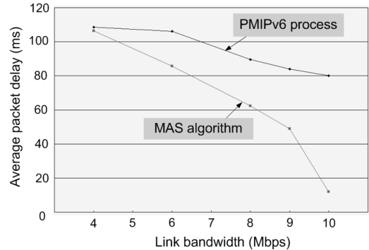
그림 10. 트래픽 로드 변화에 따른 평균 패킷 지연시간 Fig 10. Average packet delay depending on change of traffic load
