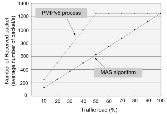
그림 7. 트래픽 로드 에 따른 받은 패킷 수 Fig 7. Number of received packets depending on traffic load
