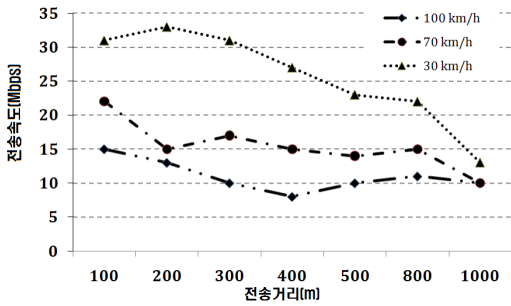
그림 3. 차량속도와 거리에 따른 전송율
