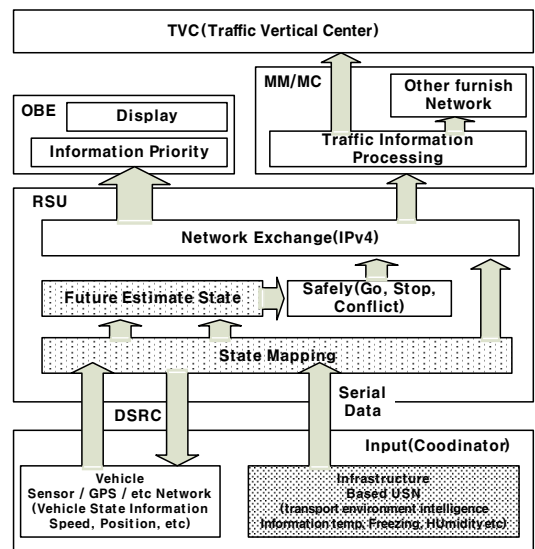
그림 2. USN과 ITS 네트워크 연동 구조
