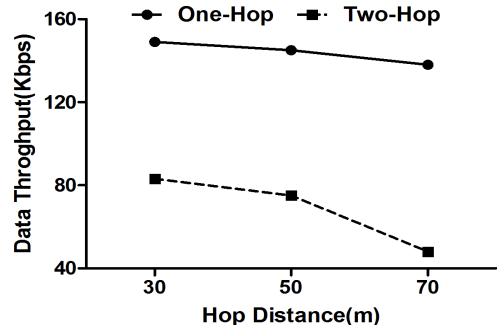
그림 5. 거리에 따른 전송 대역폭
