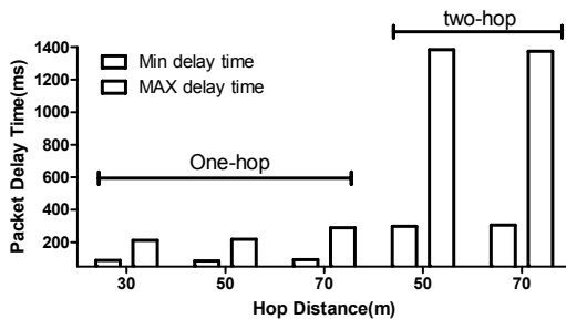
그림 4. 센서 노드의 전송 지연시간
