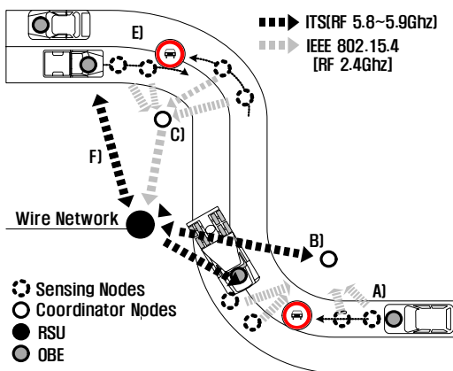
그림 1. USN과 ITS 시스템의 서비스 시나리오
