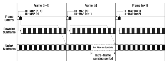
(b) FDD
