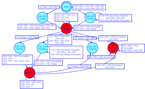
(b) 호 연결 관련 상태 천이도 예
