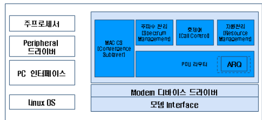
그림 3. 무선인지 단말 소프트웨어 구성
