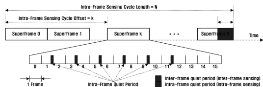
그림 4. IEEE 802.22 표준규격 Quiet Period 구간 할당 스케줄링
