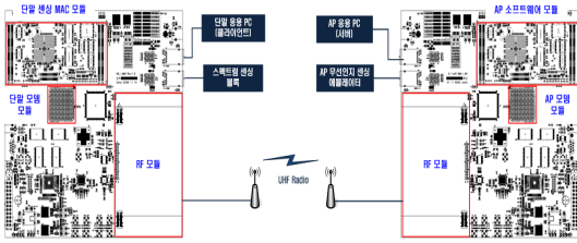
그림 10. 테스트를 위한 전체 시스템 구성도
