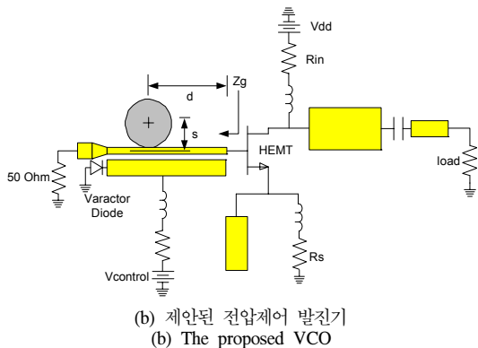
그림 2. 전압제어 발진기의 구조; (a) 일반적인 전압제어 발진기, (b) 제안된 전압제어 발진기 Fig. 2. VCO configurations; (a) the conventional VCO, (b) the proposed VCO
