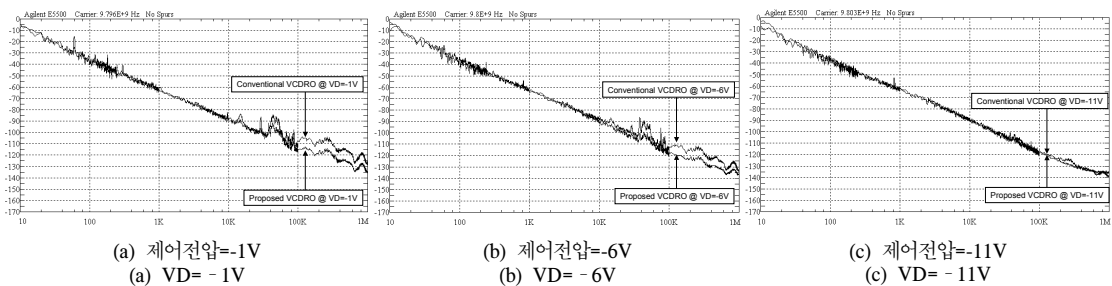
그림 6. 제안한 전압제어 발진기와 일관적인 전압제어 발진기의 제어전압에 따른 위상잡음 특성 비교; (a) 제어전압이 -1V일 때, (b) 제어전압이 -6V일 때, (c) 제어전압이 -11V일 때 Fig. 6. Measured results of the phase noise characteristics between the proposed VCO and a conventional VCO; (a) VD= -1V, (b) VD= -6V, and (c) VD= -11V.
