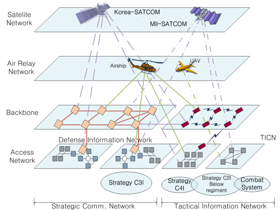
그림 1. 전술 정보 통신망 (TICN) 개념도 [4] Fig. 1. Key map of TICN [4]
