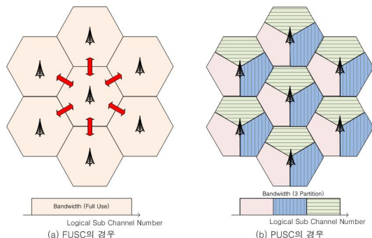
그림 3. 부반송파 할당 방식 Fig. 3. Sub-carrier allocation schemes
