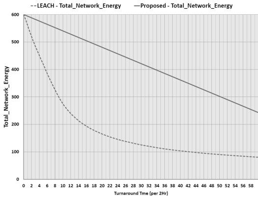
그림 6. 총 네트워크 에너지 결과 그래프
