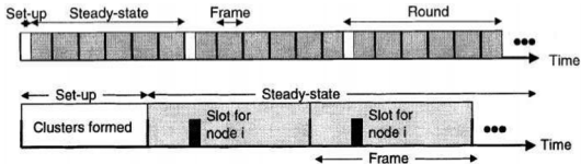
그림 1. LEACH의 타임라인(Time Line) & 구조
