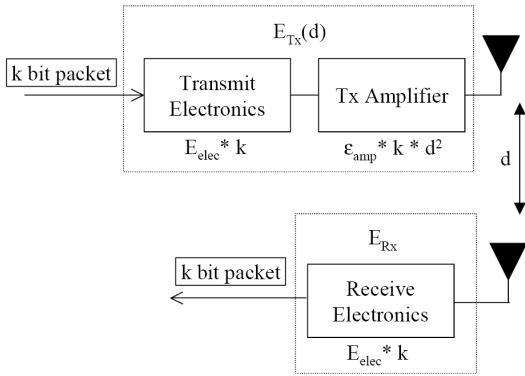
그림 5. 1:1 Data 전송 시 소비되는 에너지
