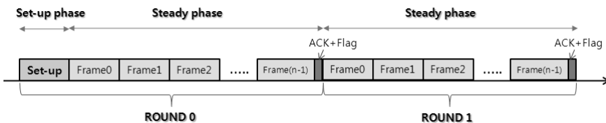
그림 4. 제안한 알고리즘의 라운드 구조
