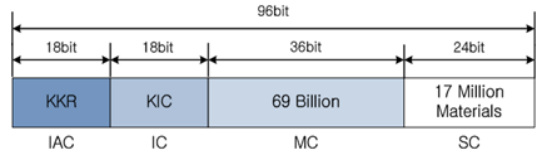
그림 2. 건설자재 정보 관리를 위한 RFID 태그 코드 체계
