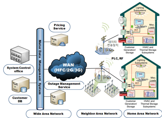
그림 1. 지능형 원격검침 시스템 구성도
