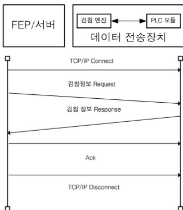
그림 4. FEP/서버 및 데이터 전송장치 간 통신절차
