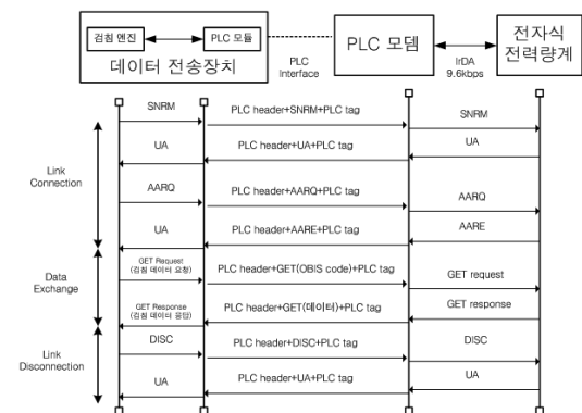
그림 3. DLMS/COSEM 기반 검침 데이터 수집 절차
