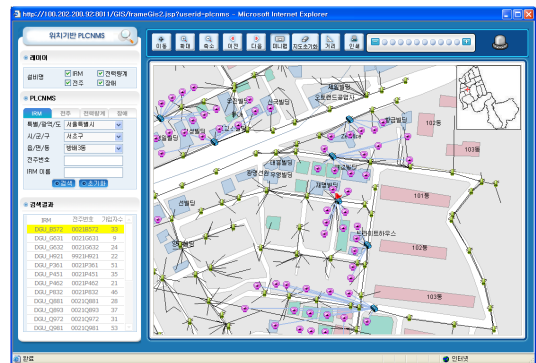
그림 5. GIS기반 NMS
