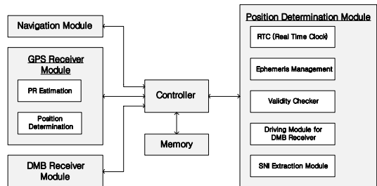
그림 3. T-DMB 와 GPS 수신기의 블록 다이어그램
