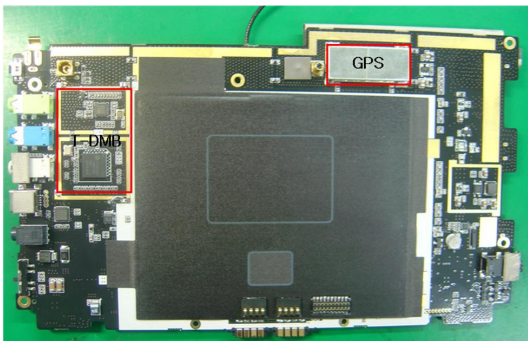
(b)보드 뒷면
