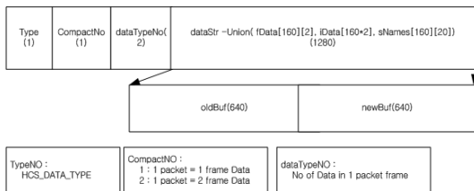
그림 6. 패킷 구조
