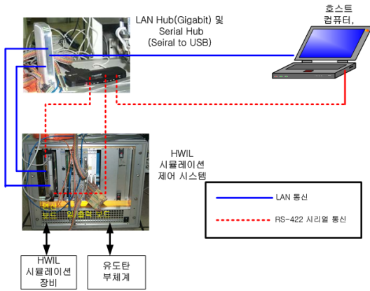
그림 2. 하드웨어 구성
