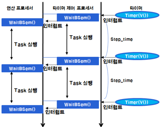
그림 3. 실시간 타이머 제어 기법
