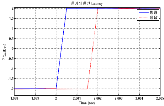
그림 12. 아날로그 통신 시간 지연
