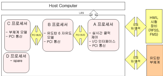
그림 8. HWIL 시뮬레이션 제어 시스템
