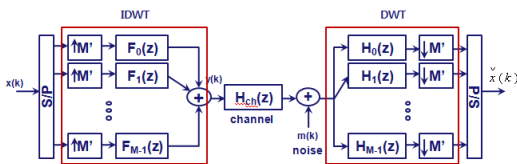
그림 1. Cosine modulated filter bank 구조
