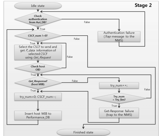
그림 6. CSCF 성능정보 추출과정(Stage 2)
