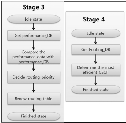
그림 7. CSCF의 성능 분석 및 결정
