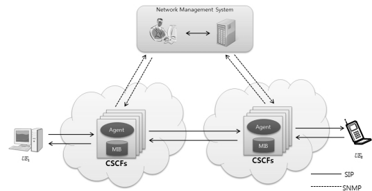
그림 1. IMS관리 시스템 구조
