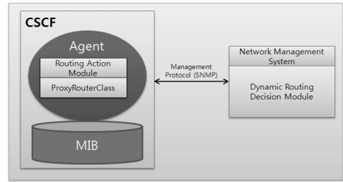
그림 3. 동적 라우팅을 위한 관리 에이전트의 구조
