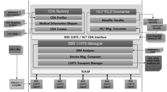
그림 5. IEEE11073/HL7 변환 게이트웨이 구조
