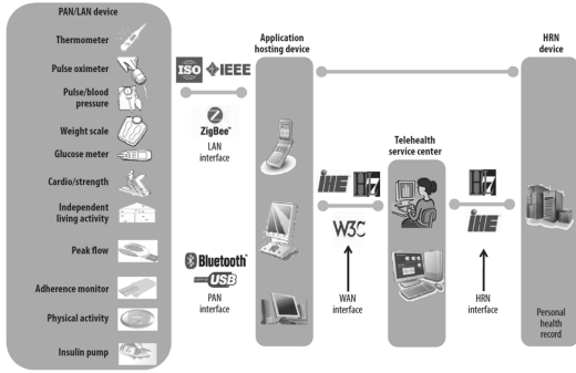
그림 3. Continua Health Alliance의 telehealth ecosystem
