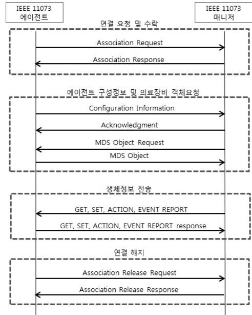
그림 6. IEEE 11073 매니저와 에이전트 간 최초 접속 및 데이터 전송 절차
