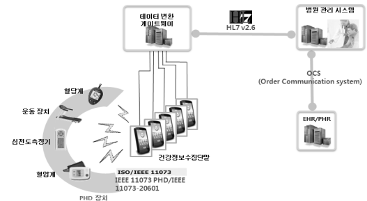
그림 4. 계층적 구조 기반 ISO/IEEE 11073과 HL7의 연동 서비스 구성도
