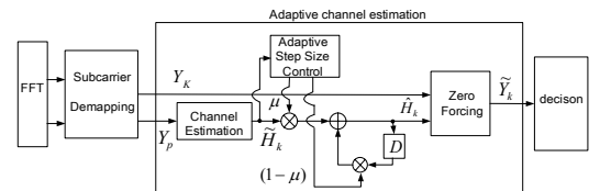
그림 6. 비선형을 고려한 적응적 채널 추정. Fig. 6. Adaptive channel estimation that consider non-linear.
