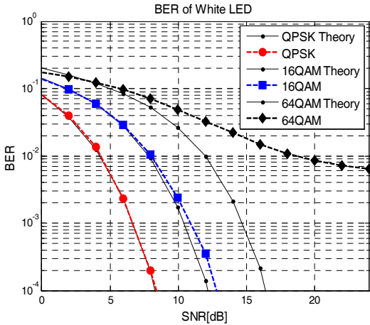
그림 3. White LED를 고려한 OFDM의 변조 방식에 따른 BER. Fig. 3. BER of white LED according to modulation type of OFDM.
