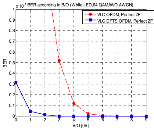
그림 8. B/O의 BER 성능 Fig. 8. BER performance according to B/O.
