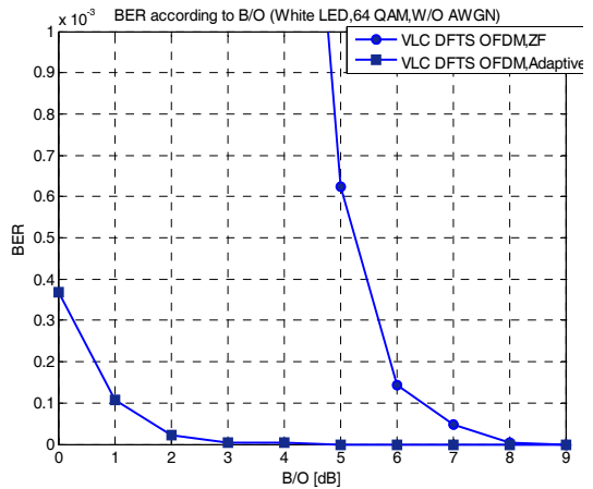
그림 9. 적응적 채널 추정의 B/O의 BER 성능 Fig. 9. BER performance according to B/O of adaptive channel estimation.
