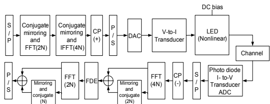
그림 5. VLC DFTs OFDM의 수신 성능 개선을 위한 시스템 Fig. 5. System for VLC DFTs's reception performance improvement
