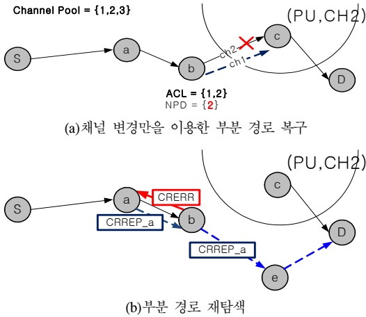
그림 6. 부분 경로 복구 및 경로 재탐색과정.
