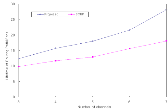
그림 9. 채널의 수에 따른 경로의 지속 시간.
