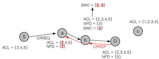
그림 5. 역방향 SWC 정보 갱신.
