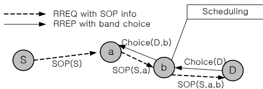
그림 1. SORP 라우팅
