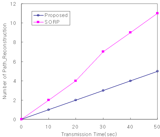
그림 10. 경로 재 설정 횟수.
