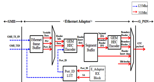
그림 6. 이더넷 정합기의 송신부의 블록 다이어그램 Fig. 6. Ethernet adaptor transmitter block diagram.
