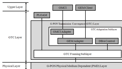
그림 1. G-PON 계층 구조 Fig. 1. Hierarchical structure of G-PON.
