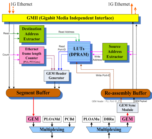
그림 5. 이더넷 정합기의 구조 Fig. 5. Structure of Ethernet adaptor.
