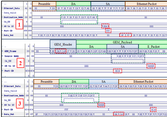
그림 14. LUT의 MAC 주소 학습 Fig. 14. MAC address learning of LUT.
