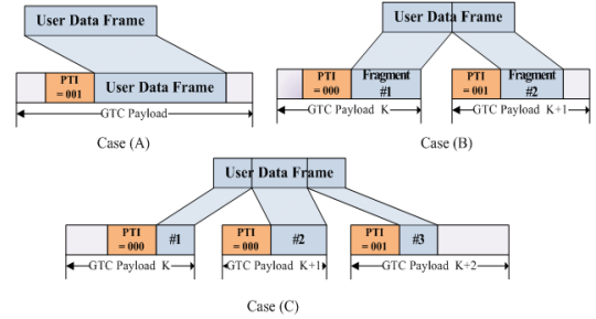
그림 3. GEM 프레임과 GTC 유료부하 Fig. 3. Payload of GTC and GEM frame.
