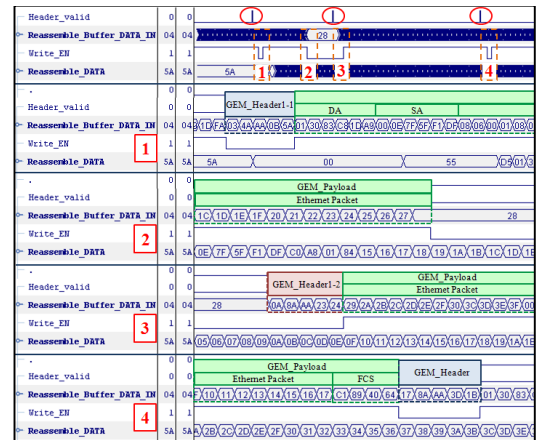
그림 12. GEM 재조립 버퍼의 입력 Fig. 12. Input of GEM reassemble buffer.
