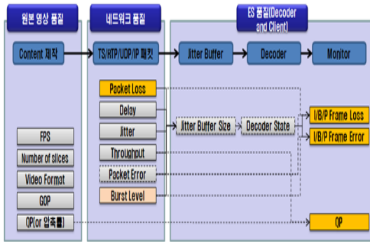
그림 5. IPTV에서 영상 미디어 전달 과정과 이와 관련된 품질 지표들
