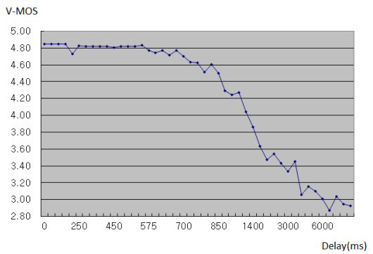
그림 7. MOS에 대한 지연의 영향
