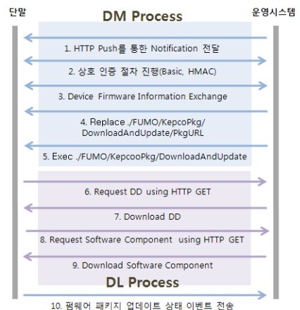
그림 5. 펌웨어 업데이트 동작 절차
