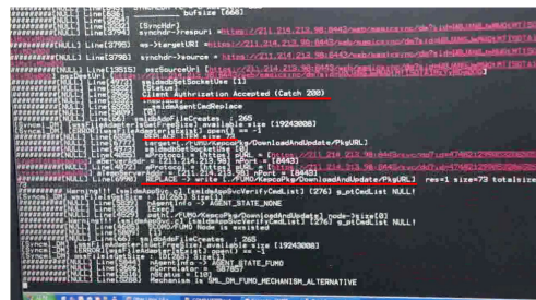
그림 7. DM 구현 예(FUMO 실행하면)
