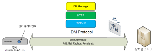
그림 1-B. 장치관리 기술 구성도
