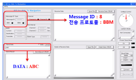
그림 8. 데이터송신 화면 Fig. 8. Program of data transmission
