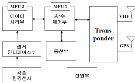
그림 2. 모듈의 하드웨어 구성도 Fig. 2. H/W diagram of module
