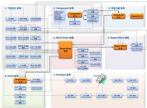
그림 5. 데이터 흐름도
