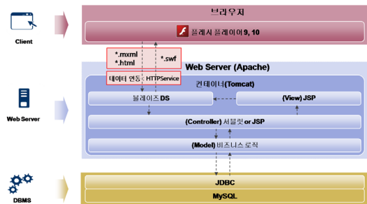
그림 3. SHERP 구현 계층
