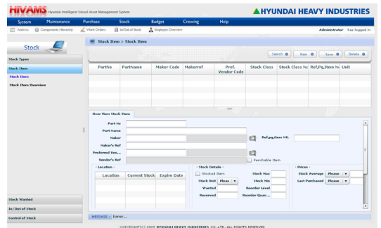
그림 14. 예비 부품 등록
