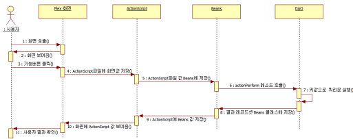
그림 9. 단위화면 실행 흐름도
