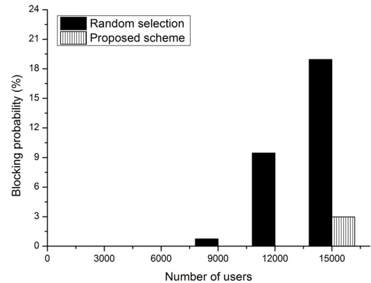
그림 7. 랜덤선택과 제안방안과의 블로킹 확률 비교
