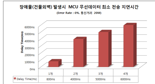
그림 17. 장애물이 있는 경우 최소 MCU 전송지연시간
