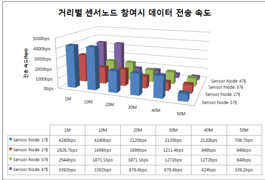
그림 18. 거리별 참여 센서노드 수에 따른 데이터 전송속도 능함을 알 수 있다.
