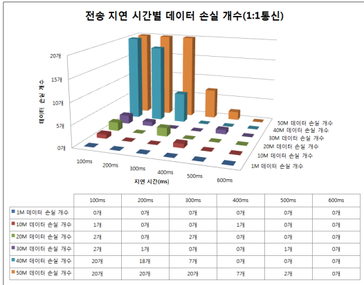
그림 13. 참여노드 1:1 데이터전송에서 지연시간에 따른 데이터 손실률 측정
