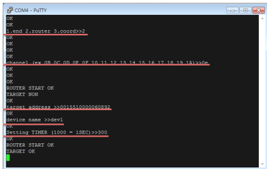
그림 3. 라우터의 설정 과정
