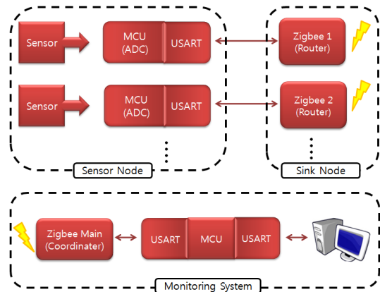
그림 1. 제안된 무선 센서네트워크의 구조
