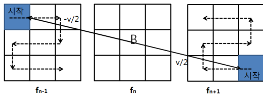
그림 2. 양방향 움직임 추정 및 보상 보간 방식
