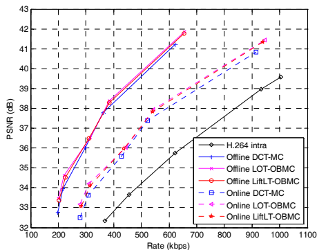
그림 9. Foreman(QCIF) 영상의 DVC 시스템에서의 R-D 성능 그래프 (key 프레임을 부호화한 경우)
