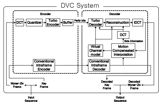
그림 1. DVC 시스템
