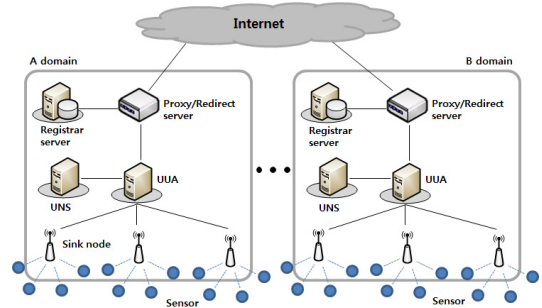
그림 2. UMS 시스템 구조
