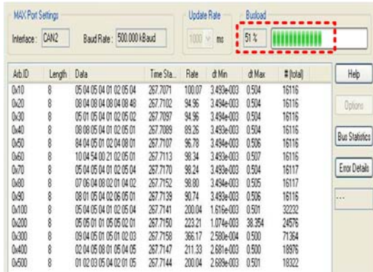
그림 5. 송신 데이터 Fig. 5. Transmission data
