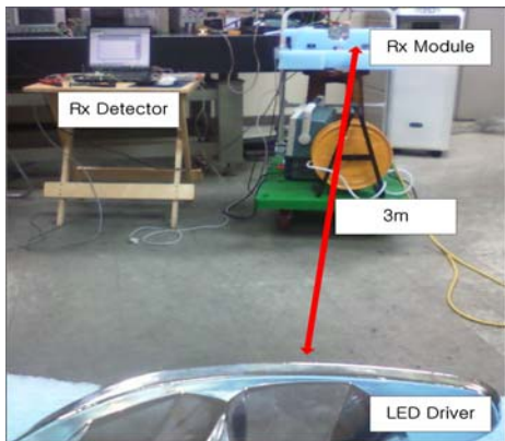
그림 3. 실험의 구성 사진 Fig. 3. Photograph of experimental setup
