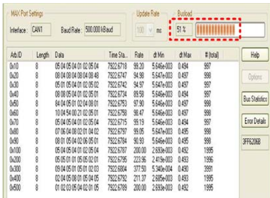
그림 6. 수신 데이터 Fig. 6. Reception data
