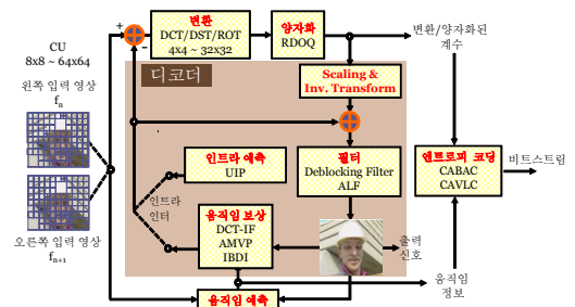
그림 5. HEVC를 이용한 양안식 영상의 부호화기 구조
