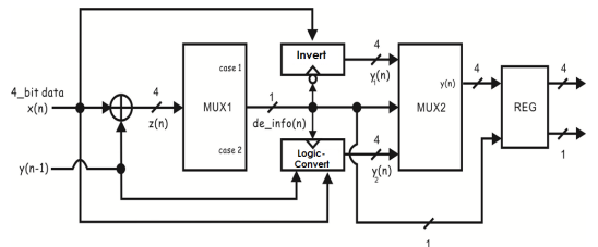
그림 2. 제안한 버스 인코딩 기법의 블록 다이어그램
