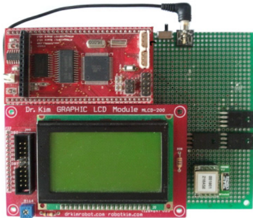
그림 6. IEEE 11073 PHD 지원 확장 모듈
