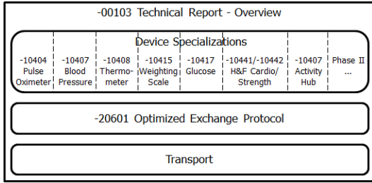
그림 2. IEEE 11073 PHD 프로토콜 구조
