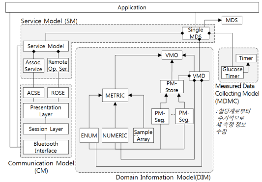
그림 7. IEEE 11073 PHD 지원 확장 모듈 소프트웨어 구조
