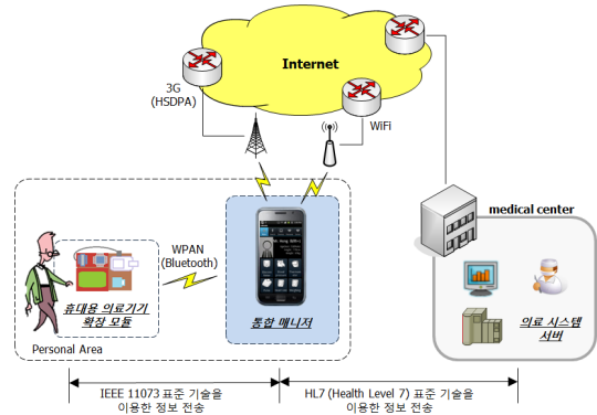
그림 4. IEEE11073/HL7 기반의 유헬스 시스템
