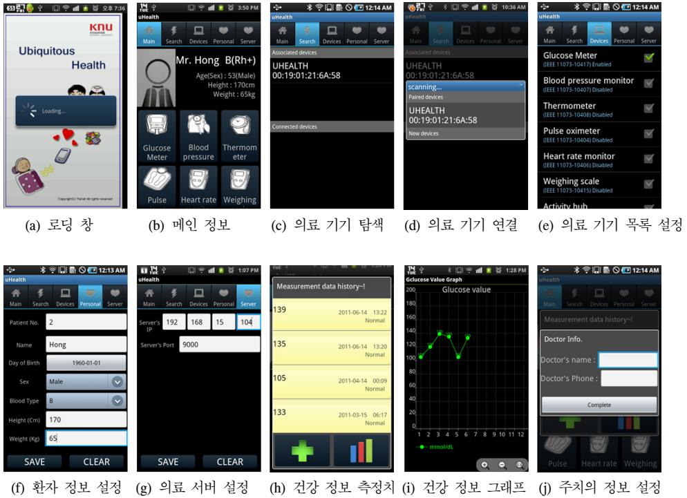
그림 10. 스마트폰 기반의 통합 매니저 GUI 화면
