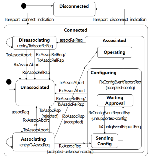
그림 3. IEEE 11073의 상태천이도
