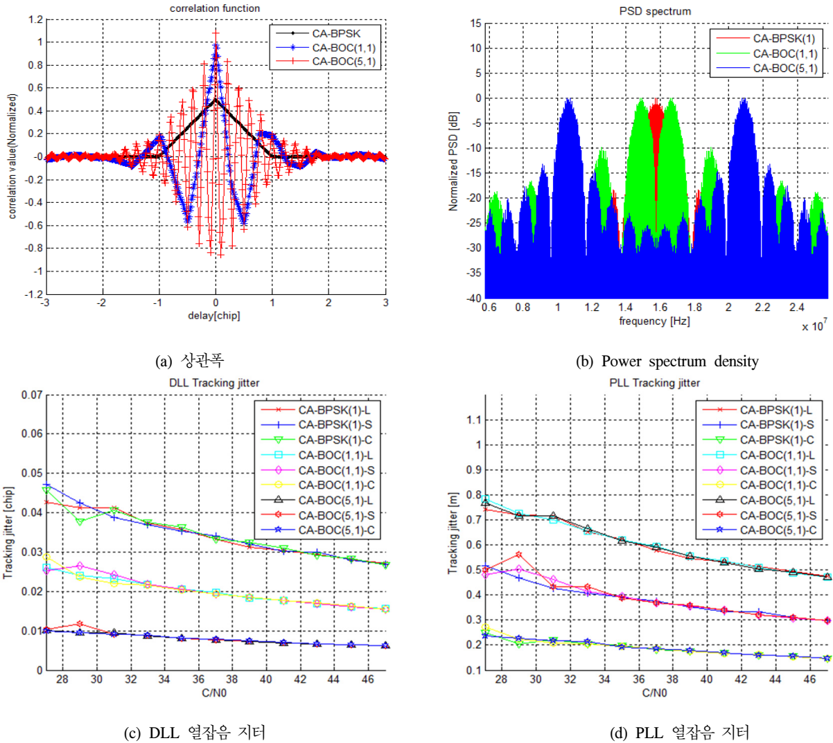
그림 2. C/A 코드 사용 시 변조기법 및 주파수 대역에 따른 수신 성능 Fig. 2. The receiver performance
