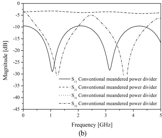
그림 5. 기존의 전력 분배기 (a) 곧은 \lambda/4 전송선의 분기경로를 갖는 전력 분배기 (b) \lambda/4 의 미앤더링 된 전송선의 분기선로를 갖는 전력 분배기 Fig. 5. Conventional L-band power dividers (a)Case 1: \lambda/4 transmission line power divider and results (b)Case 2: Meandered \lambda/4 transmission line power divider and results
