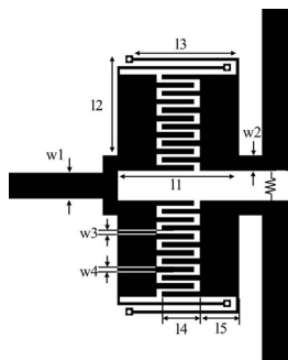
그림 6. 제안된 CRLH 0차 공진 전력 분배기 Fig. 6. The proposed compact CRLH ZOR power divider
