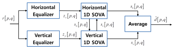
그림 2. 반복 검출 2차원 SOVA 블록다이아그램. Fig. 2. Block diagram of iteratively detecting 2-dimensional SOVA
