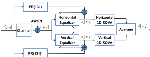
그림 1. 2차원 SOVA 블록다이아그램 Fig. 1. Block diagram of 2-dimensional SOVA
