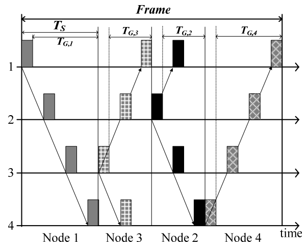
그림 2. AGT-TDMA 기법의 프레임 구조 예제 Fig. 2. Example frame structure of AGT-TDMA scheme
