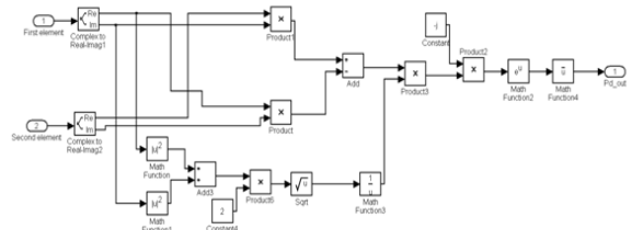
그림 4. 디지털 위상 검출기와 위상 공액기의 시뮬링크 블록도 Fig. 4. The simulink block diagram of digital phase detector and phase conjugator.
