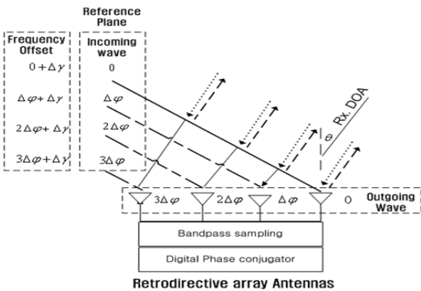
그림 2. 디지털 역지향성 안테나의 개념도. Fig. 2. The concept of digital retrodirective array antennas.
