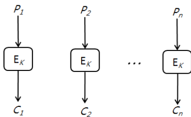
그림 1. ECB 모드 Fig. 1. ECB mode
