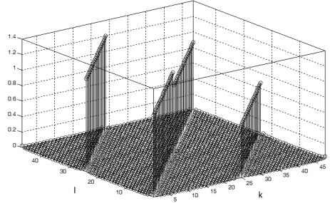
그림 1. ITU-R Ped A 2 \times 2 채널의 |h_{\text{eff},lk}| Fig. 1. |h_{\text{eff},lk}| of 2 \times 2 ITU-R Ped A channel
