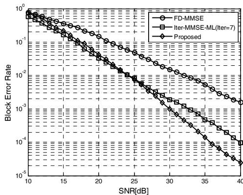
그림 2. 주파수영역 선형등화기법(FDE), 신뢰도 기반 반복적 검출기법(Iterative 반복횟수:7), 제안된 기법(proposed)의 오류성능 비교 Fig. 2. Comparison of error performance of frequency domain linear equalization (FDE-MMSE), reliability-based iterative detection (Iter-MMSE-ML, number of iterations=7), and the proposed technique.
