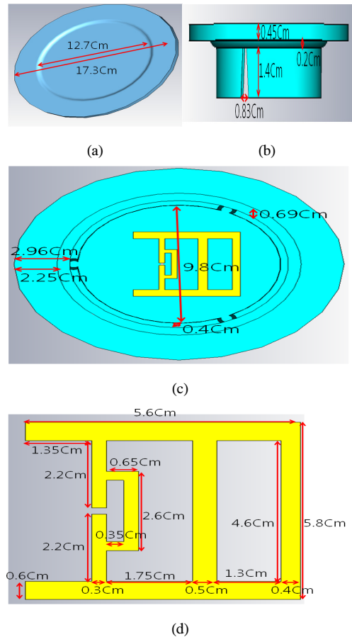
그림 1. (a) 초밥용 접시의 윗면 (b) 초밥용 접시의 옆면 (c) 초밥용 접시의 윗면과 태그 (d) 부착한 UHF 태그 Fig. 1. (a) Top view of dish, (b) Side view of dish, (c) Bottom view of dish and tag, (d) Parameters of attached Tag
