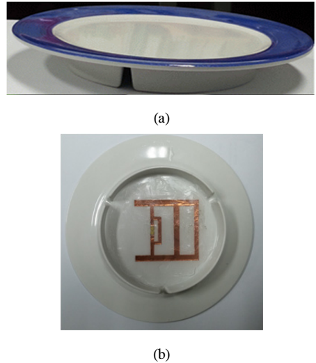
그림 2. 제작된 초밥용 접시의 UHF RFID Tag가 부착 된 (a)윗면 및 (b) 밑면 Fig. 2. (a) Top view of the dish, (b) bottom view of the dish with fabricated UHF RFID Tag
