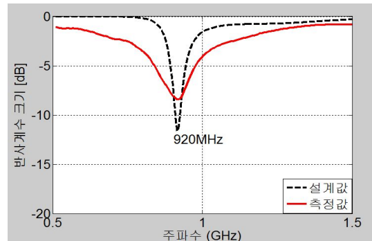
그림 3. 초밥용 접시 UHF RFID Tag 안테나의 simulation과 측정된 반사계수의 주파수별 크기. Fig. 3. Simulated and measured S11 of the fabricated UHF RFID tag on the dish.
