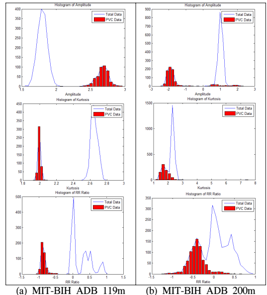
그림 3. MIT-BIH 119m 레코드와 200m 레코드의 V , K , RR 의 히스토그램 Fig. 3. Histogram of V , K , RR of MIT-BIH 119m record and 200m record.
