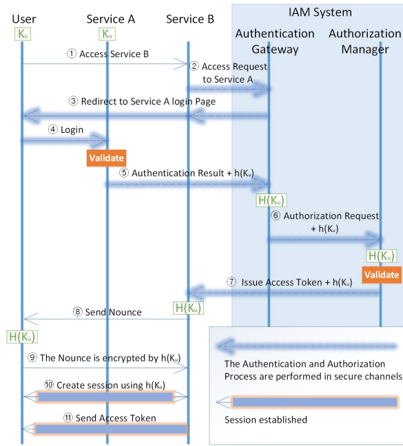
그림 2. Inter-Cloud 인증 플로우 Fig. 2. Authentication Flow for Inter-Cloud
