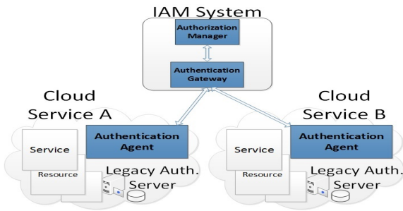
그림 1. Inter-Cloud IAM 아키텍처 구성도 Fig. 1. Inter-Cloud IAM Architecture Diagram
