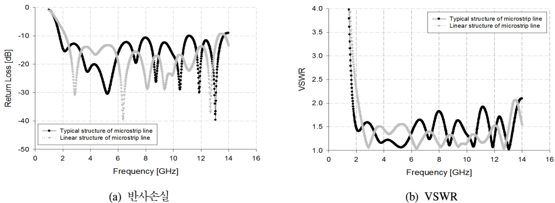
그림 2. 제안된 안테나의 반사손실 및 정재파비 예측 결과 Fig. 2. Return loss and VSWR simulation results of the proposed antenna
