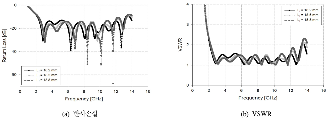
그림 3. L_f 변화에 따른 반사손실 및 정재파비 예측 결과 Fig. 3. Return loss and VSWR prediction result due to changes L_f
