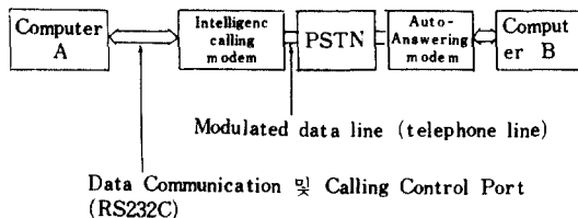
그림 2 Dial-up UUCP를 위한 hardware confiduration
