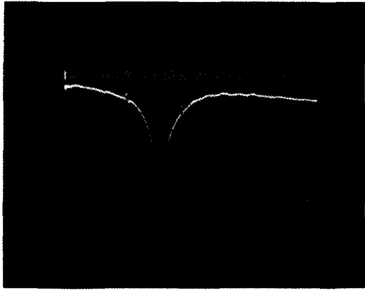
그림 2 9.9[GHz]共振器에 대한 反射損失測定值 Measured return loss as a function of frequency for 9.9GHz resonator. (V: 5dB/div, Sweep freq. 8~12GHz H: 400MHz/ div.)
