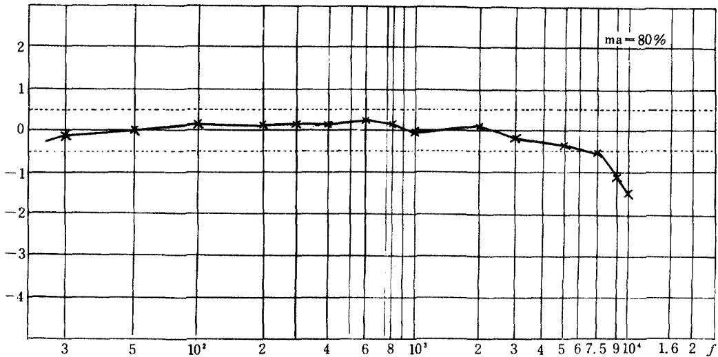
그림10 변조出力周波數特性
