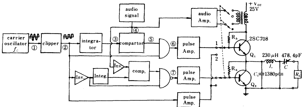
그림 7 스위칭 모드變調回路
