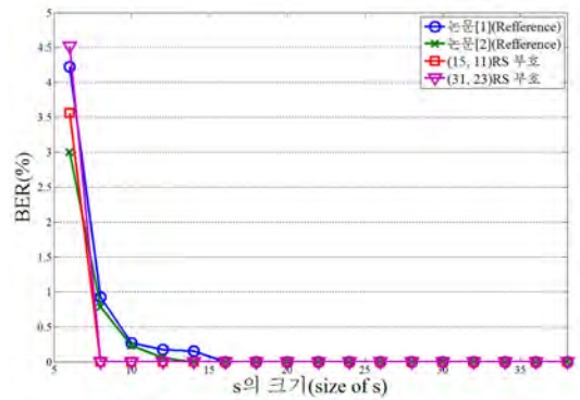
그림 4. 레나를 사용하였을 때 BER 성능 Fig. 4. BER performance when Lenna image is used
