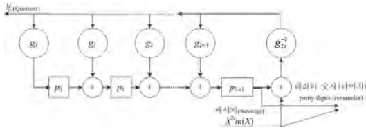
그림 2. RS 부호의 부호화 알고리즘 Fig. 2. Encoding algorithm of RS code
