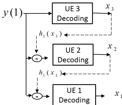
그림 2. 사용자가 3명일 때 UE-1의 송신기에서 SIC 적용 예 Fig. 2. Example of SIC for 3 Users at UE-1 Receiver
