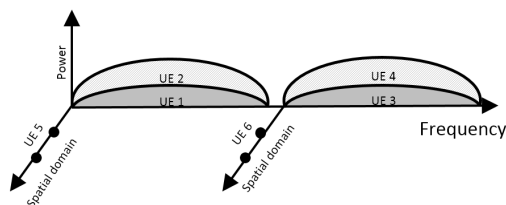
그림 5. 사용자가 6명일 때의 Spatially Modulated NOMA의 주파수 영역 Fig. 5. Frequency Band of Spatially Modulated NOMA for 6 Users
