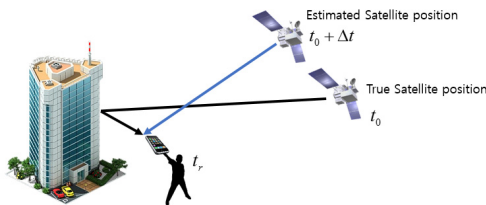
그림 3. 제의사거리 역추정 알고리즘 개념도 Fig. 3. Conceptual diagram of Pseudorange inverse estimation algorithm
