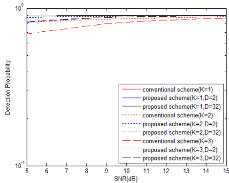
그림 3. 검파 확률 성능 비교 Fig. 3. Comparison of detection probabilities
